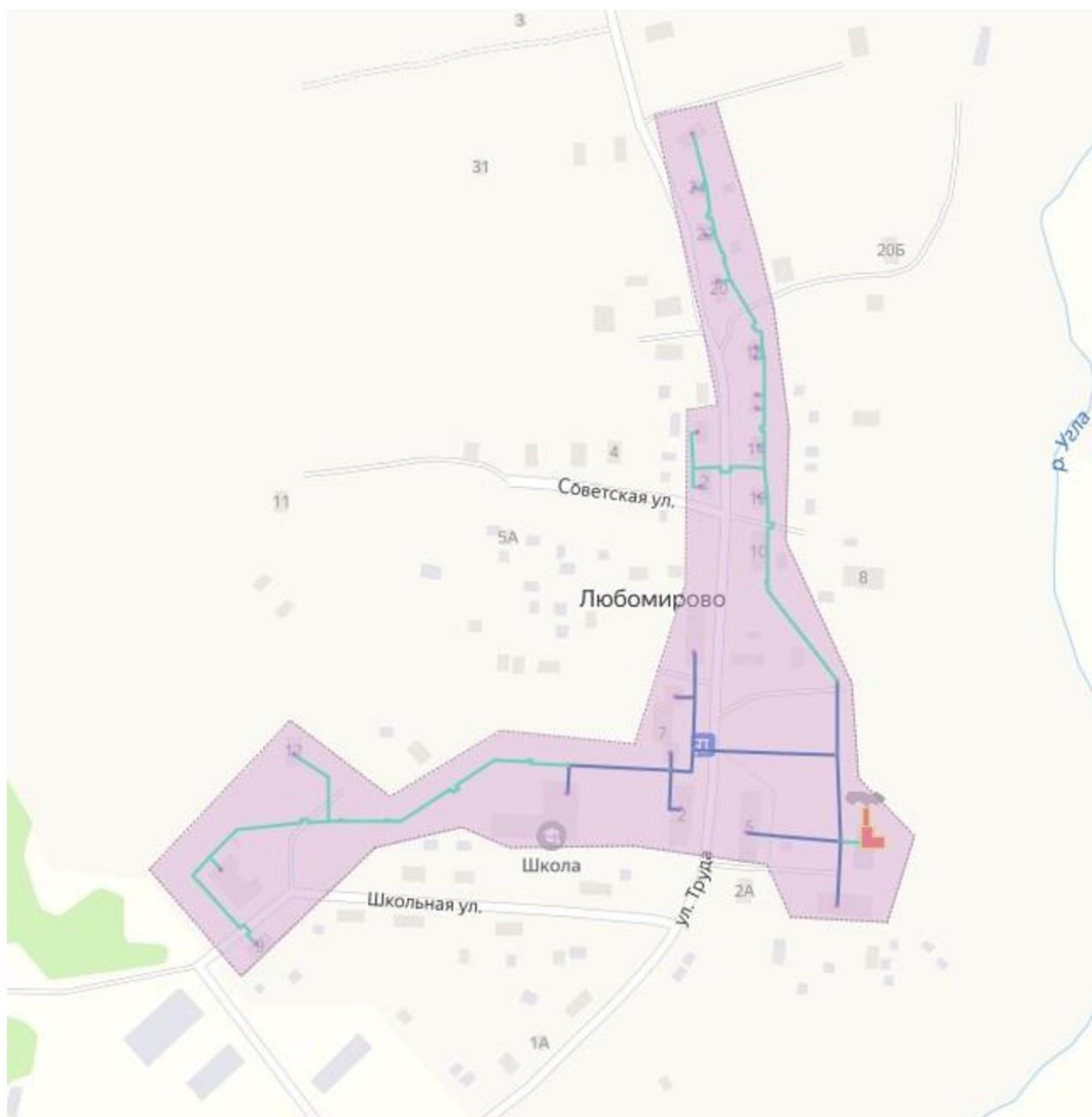
Схема тепловых сетей от котельной с.Любомирово
