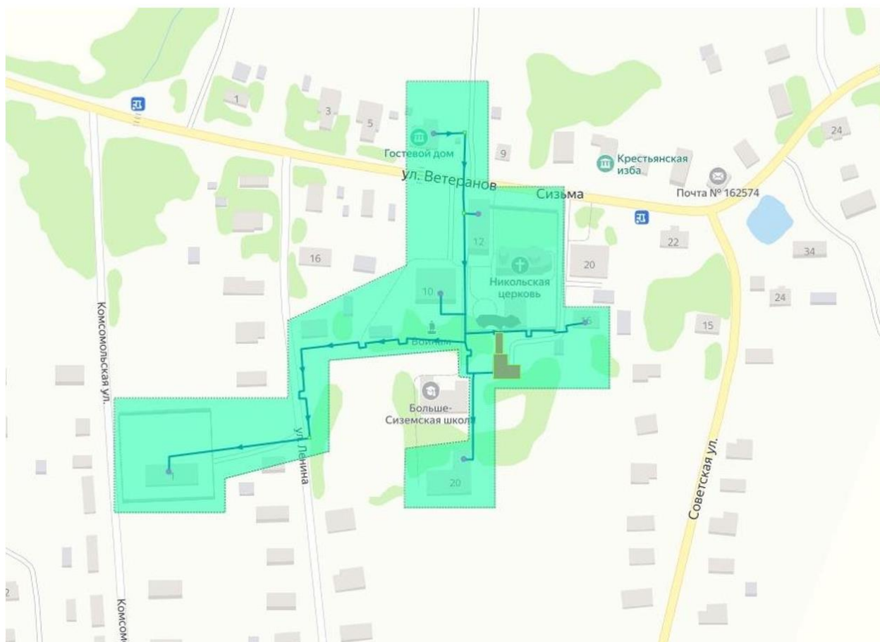
Схема тепловых сетей от котельной УК Сизьма
