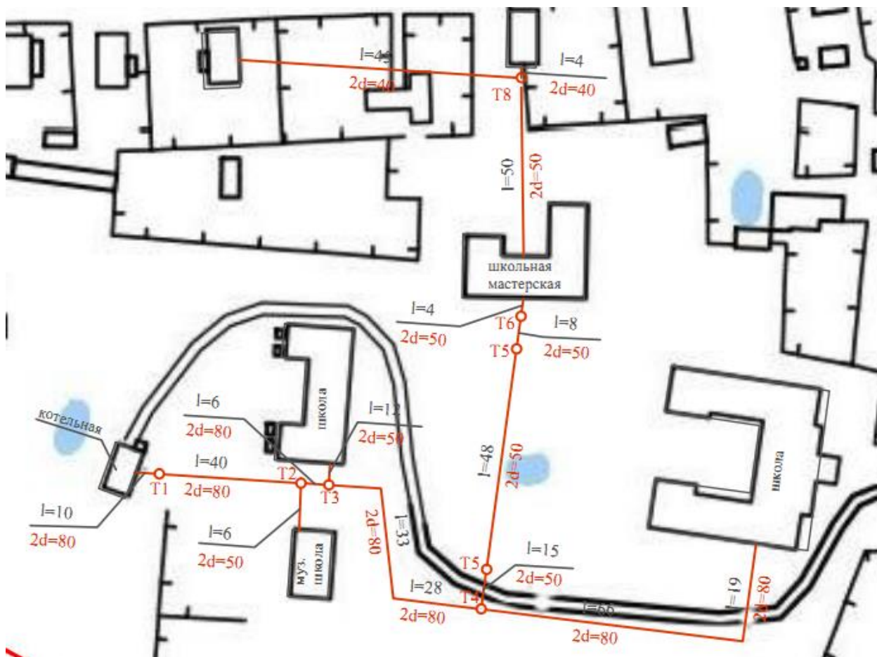
Схема тепловых сетей от котельной Школьная, п.Чебсара, пер.Краснораменский,
