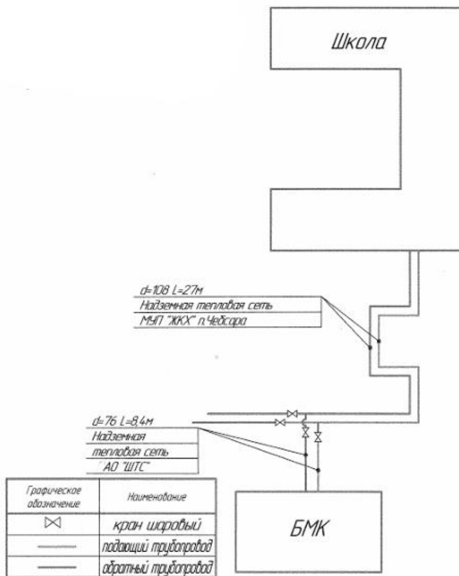
Схема тепловых сетей от котельной котельная, п.Чибсара, ул.Мира, д.27
